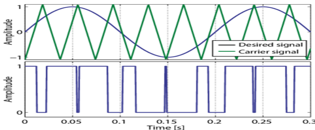
Fig. 10. PWM (Sinusoidal)
